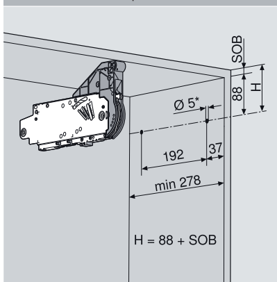
Posició tacs encastrats per mecan.
