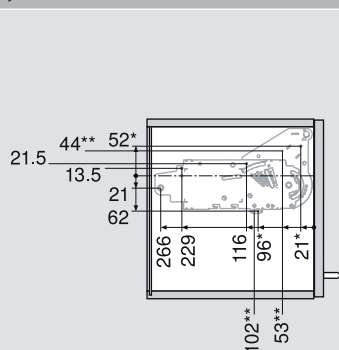
Fijació mecanisme elevació
